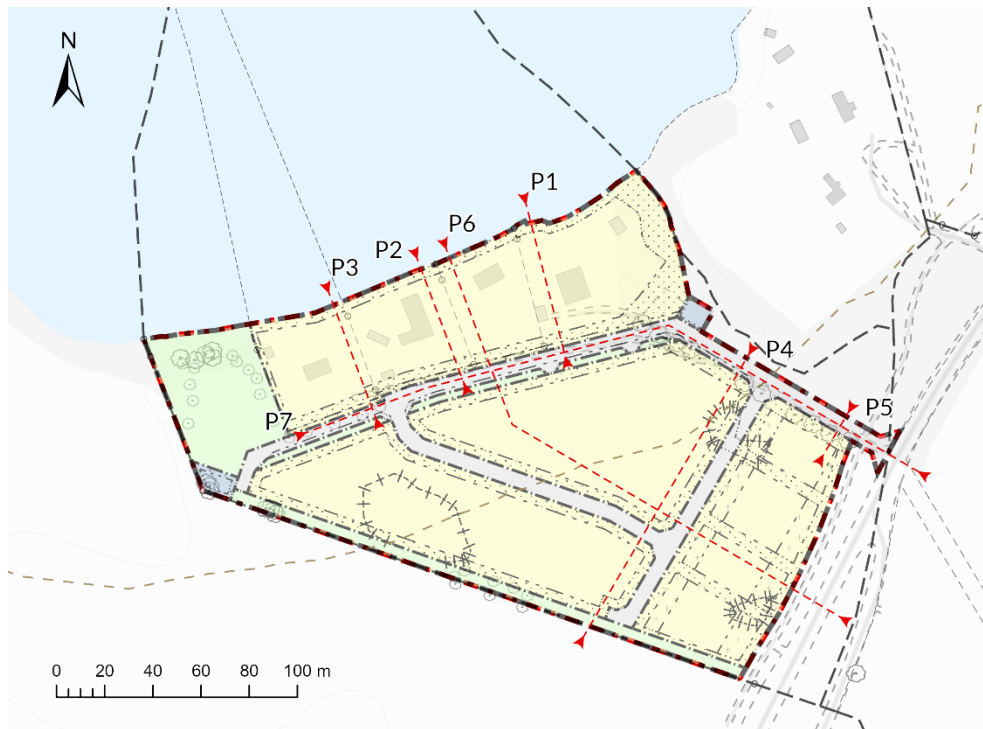
Figur 16: Markprofilinjer
